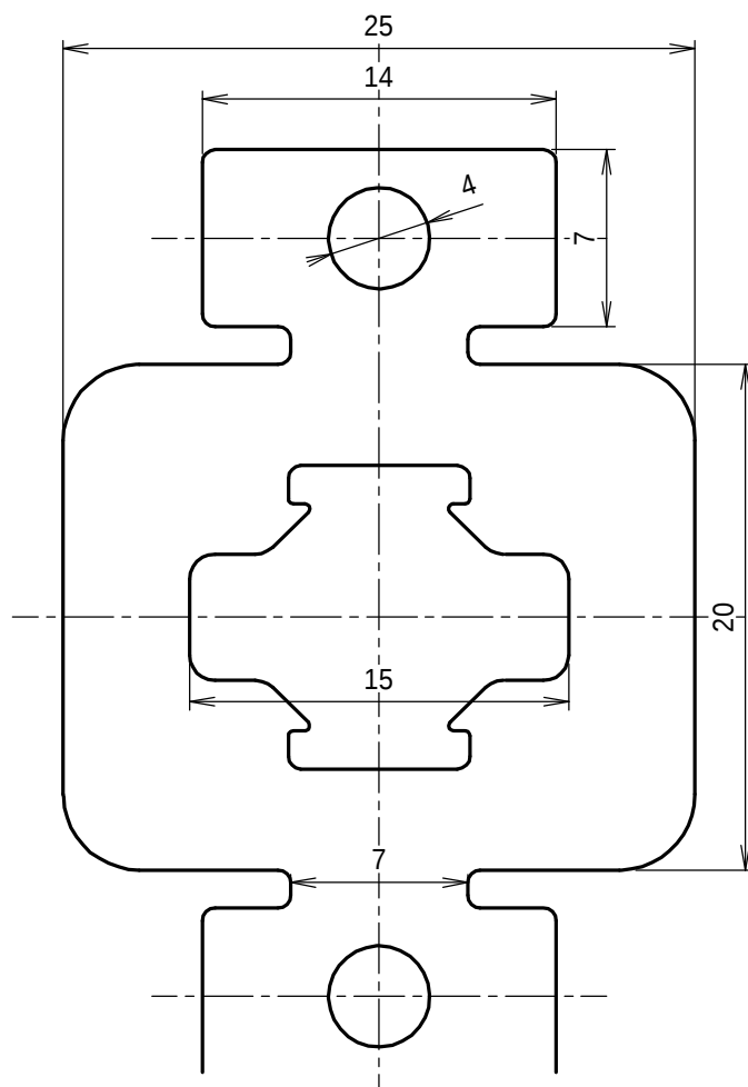
A部詳細図(3/1)
